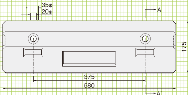
■平面図
