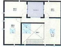
2F平面図
