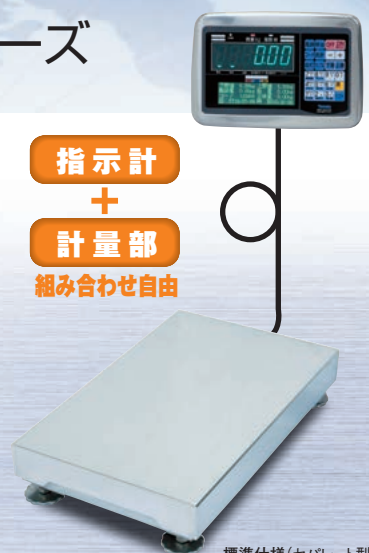
標準仕様(セ/バレート型) ※卓上型除く
