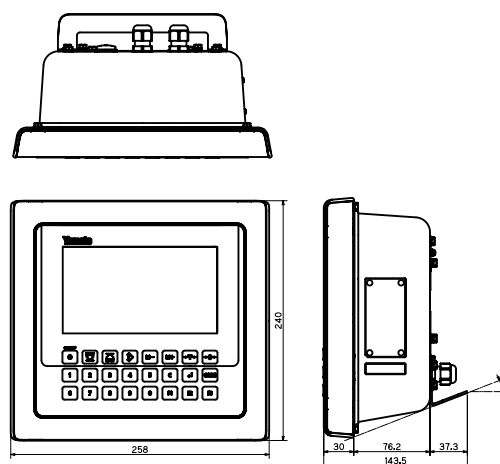
外形寸法
