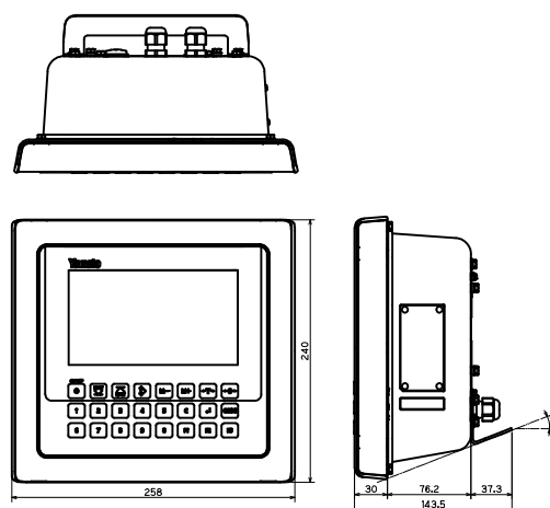
外形寸法
