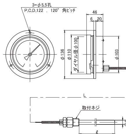
図面 ⑤ LD-100S
