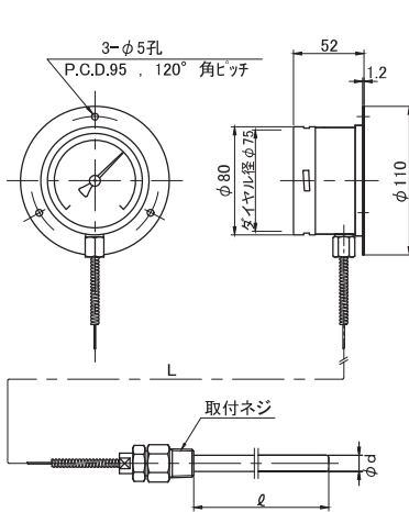
図面 ① LB-75S
