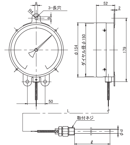
図面 ③ LB-150S
