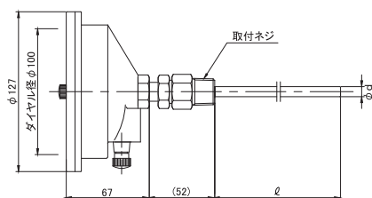
図面 ③⑬ BM-T-100E
