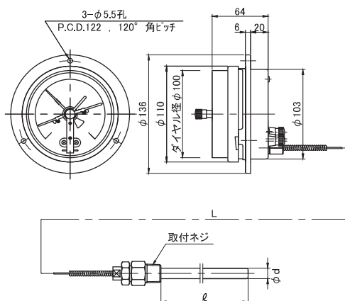
図面 ⑭ LD-100SE
