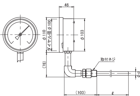
図面 ⑦ LAL-100S
