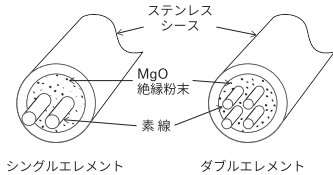
○参考構造図
