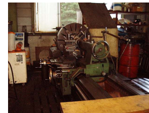
12尺旋盤 1000φ X 200 800φ X 3500
