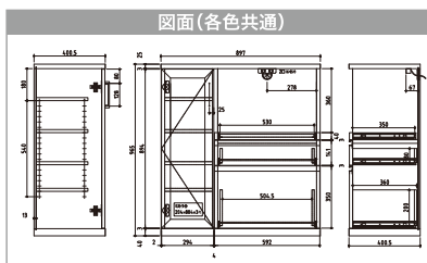
TRB-900CW
