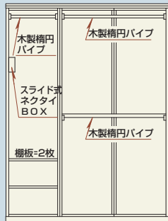
1500スライド(3枚扉) ※150幅は2BOX(3分割・ スパークアップ)になります。
