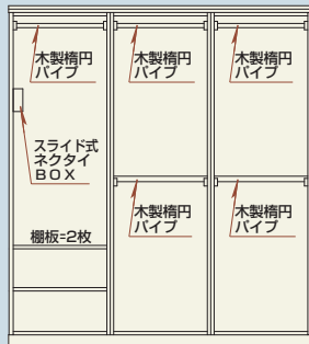
1800スライド(3枚扉) ※160幅から180幅までは 3BOX(3分割)になります。
