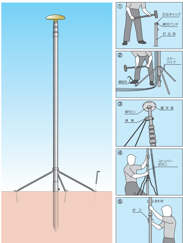
【構成】ポール・打込杭・打込キャップ・締付バンド・支柱(ステーパーパイプ)・補助杭・滑車・ロープ・ボス押え金具・扁平球
