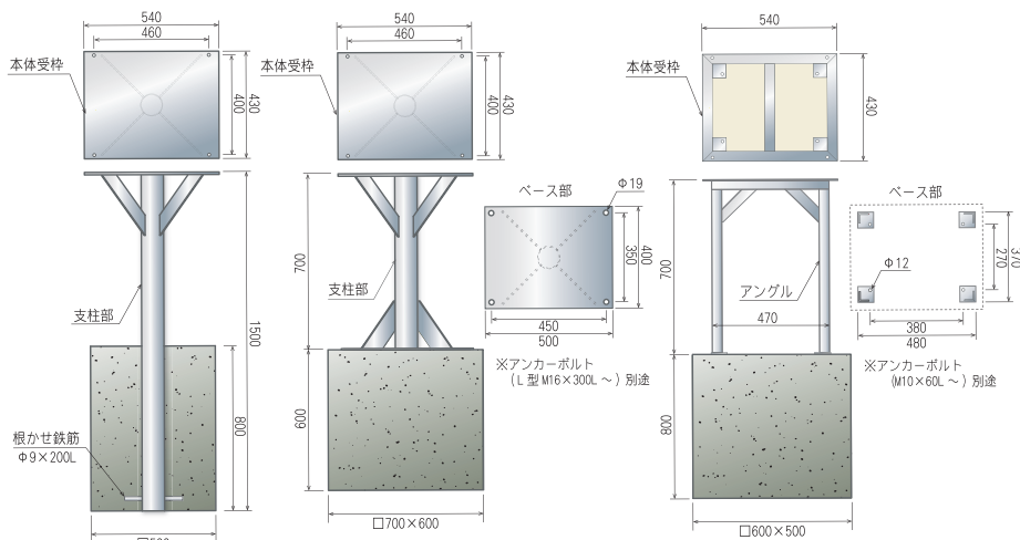
■基礎埋込用架台 SBKP01
