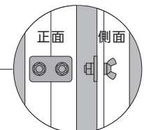
ジョイント金具・蝶ボルト
