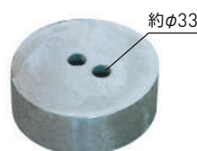
CW-04 ○約φ280×H90mm ○質量/13kg
