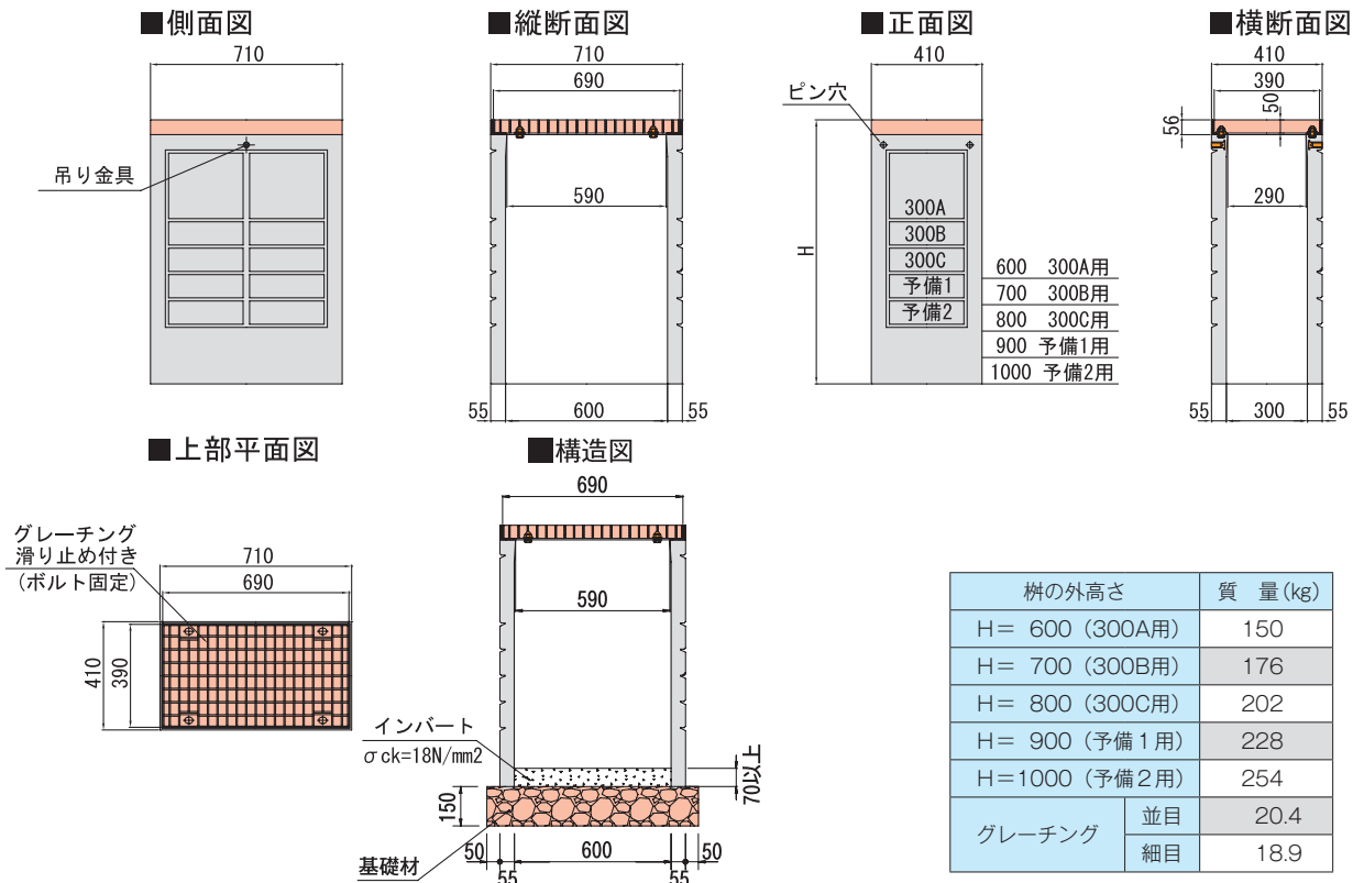
ニューパワー側溝300PML構造図
