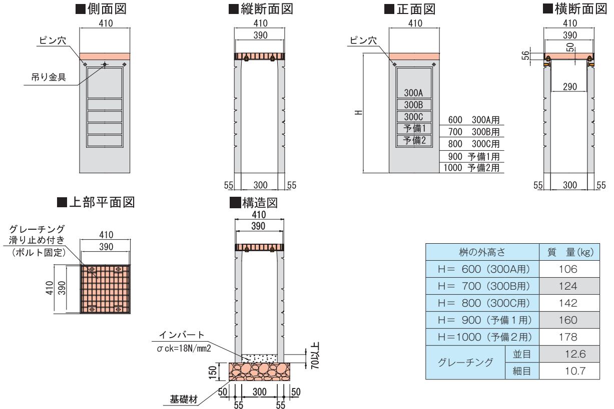
ニューパワー側溝300PML構造図
