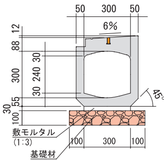
■中央断面図
