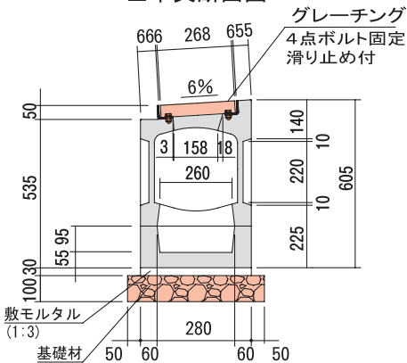
■中央断面図
