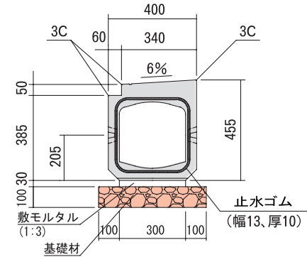
■端部断面図
