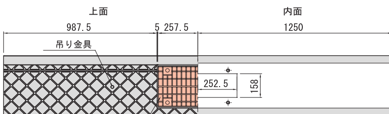
■平面図
