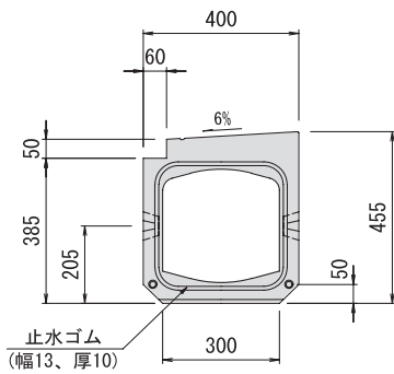
■ 端部正面図
