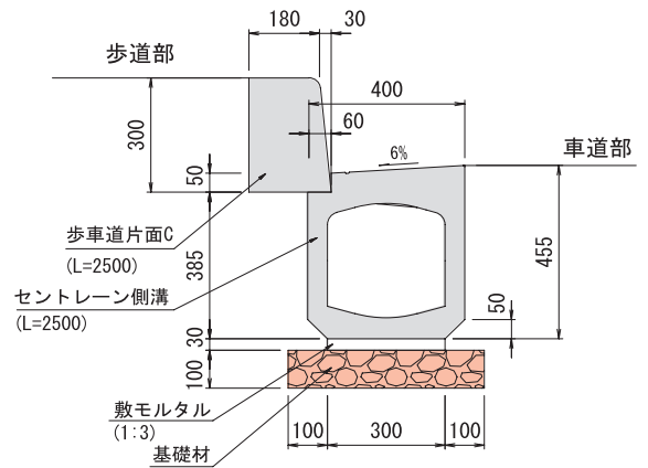
■ 側面図
