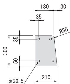
■ 端部正面図
