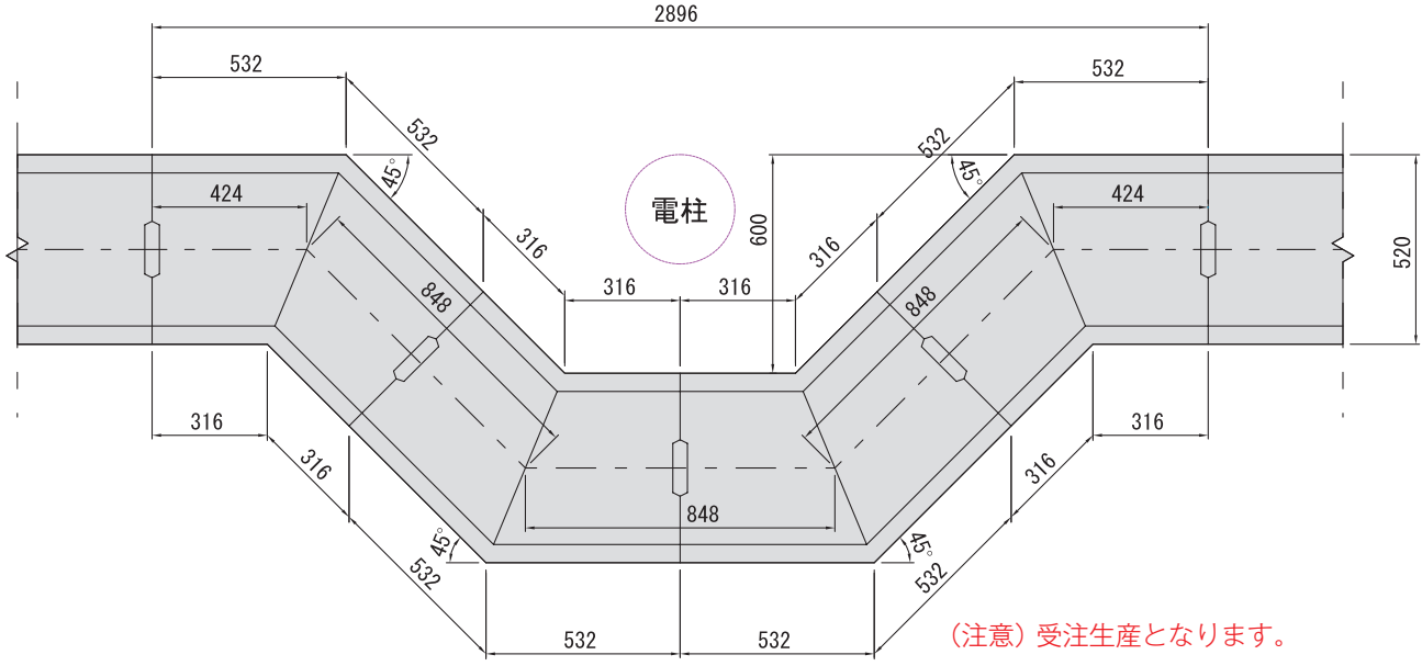
■蓋部平面図
