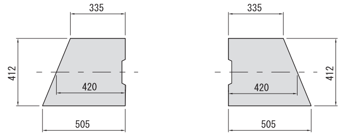
■蓋部平面図
