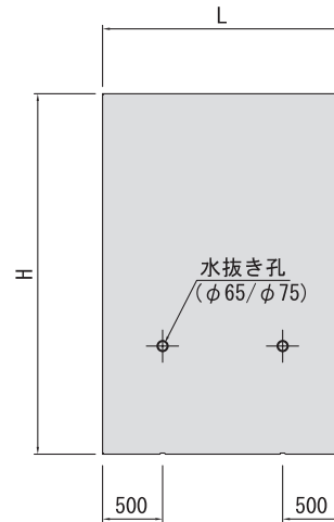
■正面図
