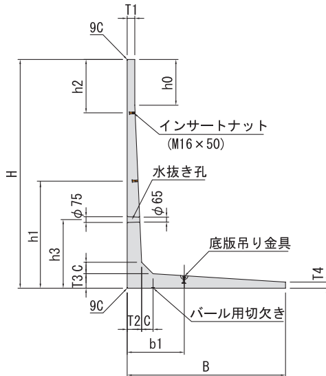
■断面図
