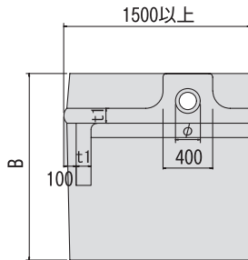
■端部用 (左)
