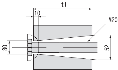
■取付詳細図
