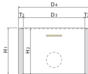
■管取付壁
