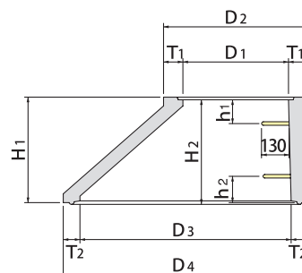
■斜壁
