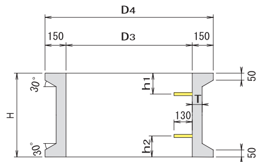
■ 断面図
