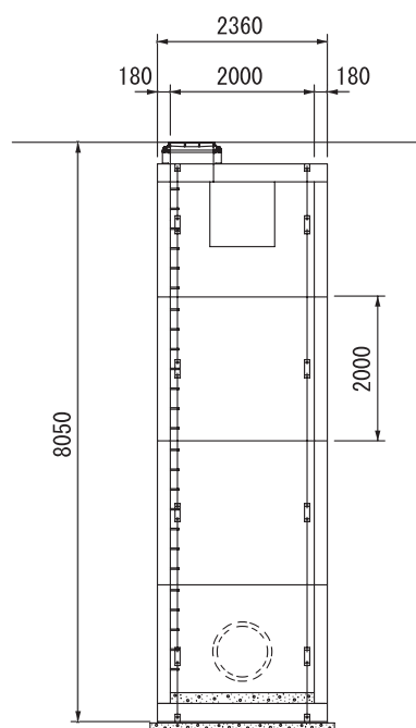
■縦断面図
