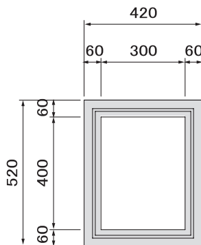
■①—①断面図
