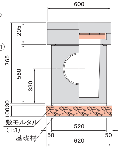
■縦断面図
