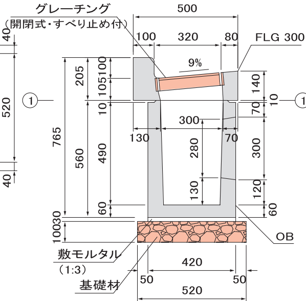
■横断面図
