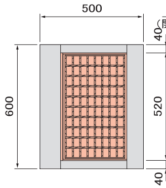
■平面図
