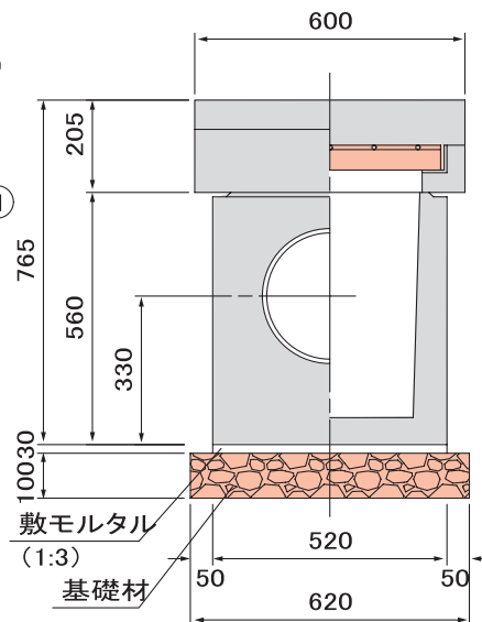
■縦断面図
