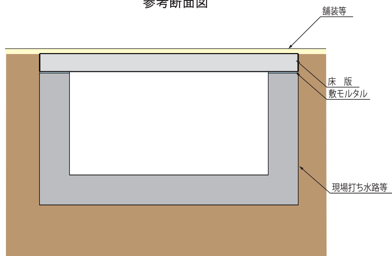
参考断面図
