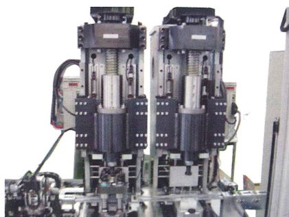
ダブルヘッドサーボプレス装置
