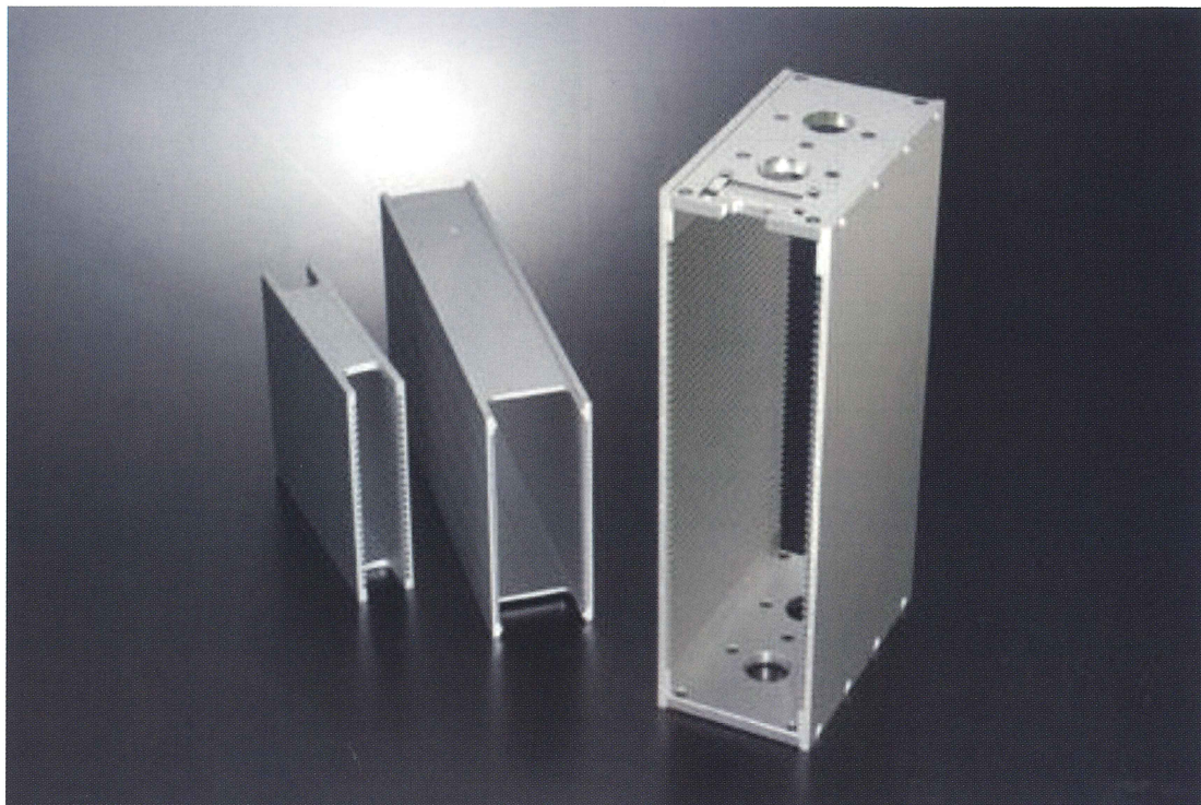
組立作業用マガジンラック(アルミ押出一体マガジン、オーダメイドマガジン)
