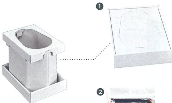
〈紙製便器 組立時〉 (耐荷重 200kg ※等分布)
