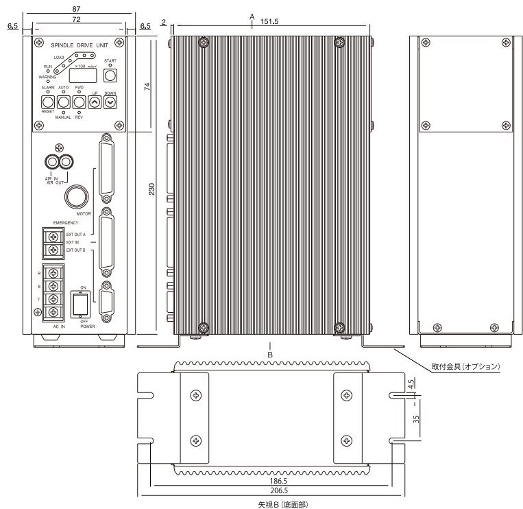
<M3コントローラー 外観図>
