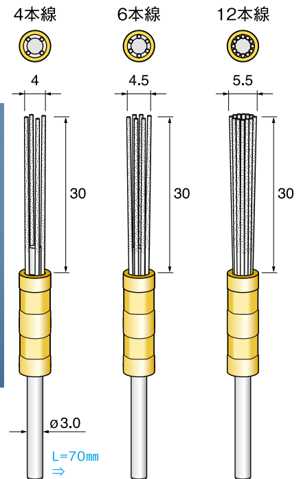
電着ダイヤモンド ワイヤーラップ Diamond Wire Lapping Tools
