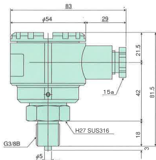
4~20mA式
