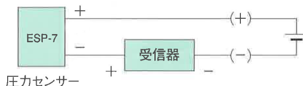
4～20mA式
