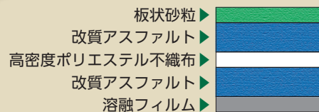
製品構造
