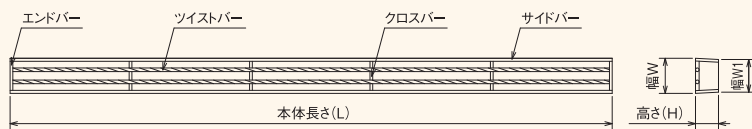
●GAK図面
