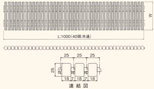
RG-S／直線タイプ連結図(1m)
