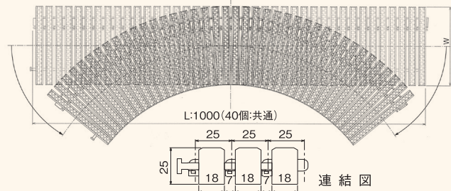
RG-R／曲線タイプ連結図(1m)
