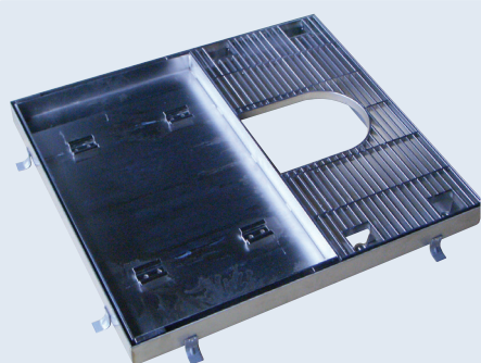
R加工／ボルト固定式グレーチング
