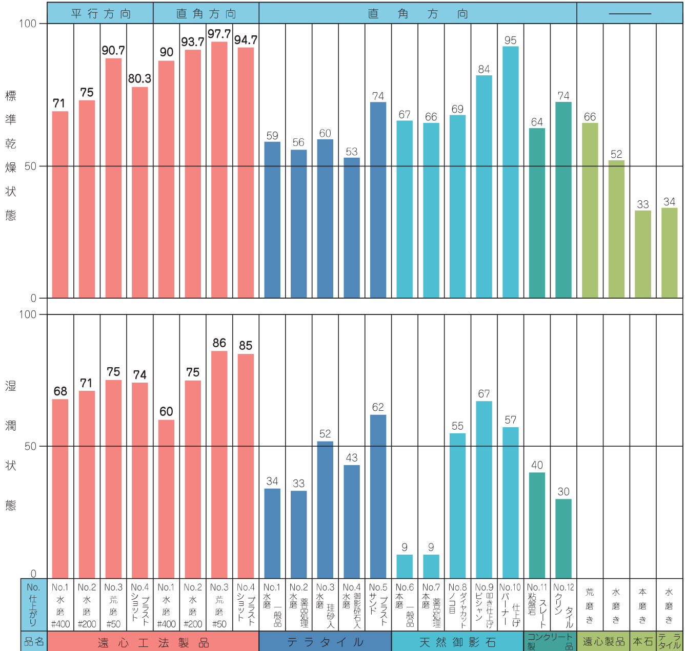
●すべり試験結果 1、2 グラフ 試験方法 ASTN303、JISA1407
