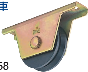
ロタ・ステンレス 重量戸車
