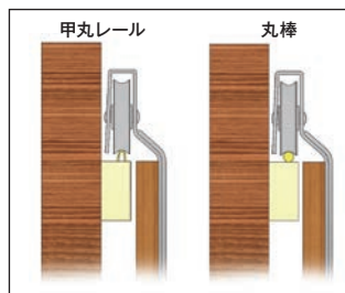
吊戸車 甲丸レール・丸棒 使用例
